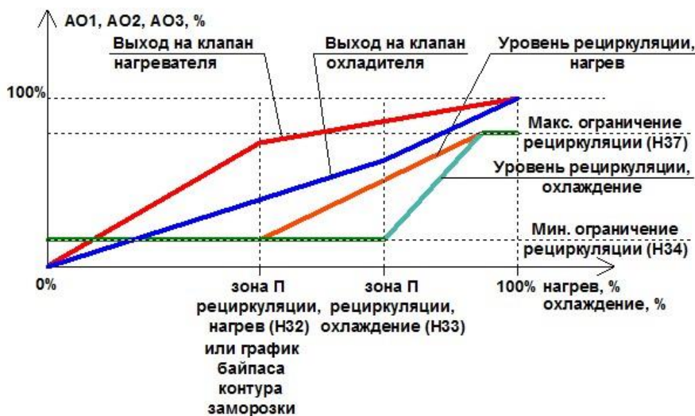
Рис. 12. Работа рециркуляции в автоматическом и ручном режиме.
