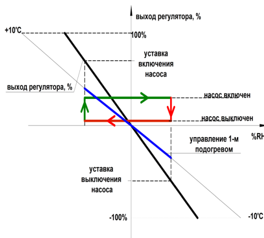
Рис. 13. График работы форсуночного увлажнителя.
