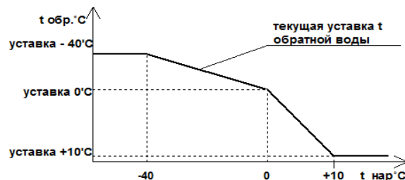
Рис.4. График текущей уставки t_{обр.} при работе вентилятора.
