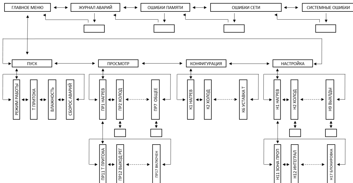
Рис. 15. Структурная схема меню контроллера RX500-V
