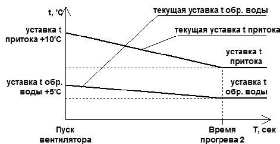
Рис.5. График работы прогрева 2 и 4 при пуске.
