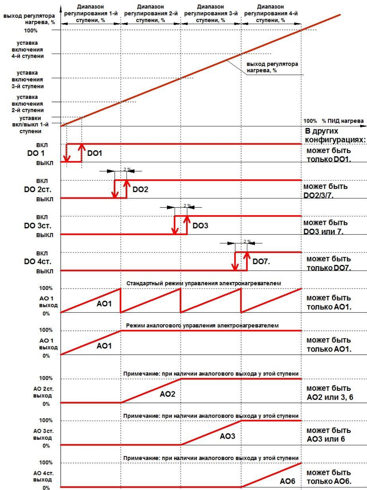
Рис. 3. Логика работы 4-хступенчатого электронагревателя.
