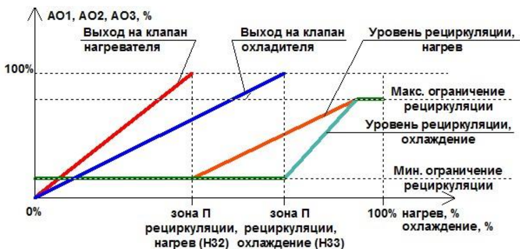
Рис. 11. Работа рециркуляции в прямом режиме.
