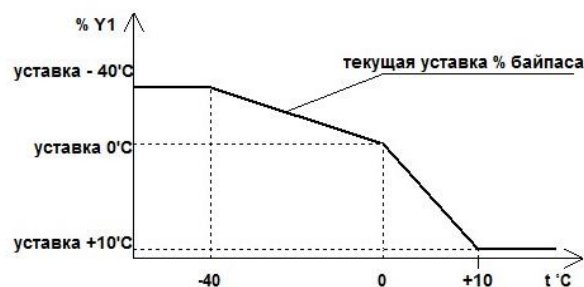
Рис. 6. График работы байпаса в автоматическом режиме.
