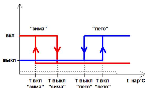
Рис. 7. График переключения климата в автоматическом режиме.
