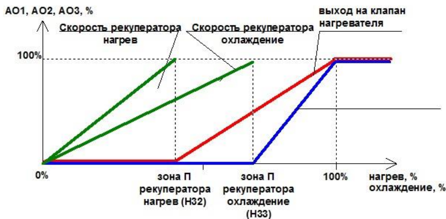
Рис. 9. Работа роторного рекуператора в прямом режиме.
