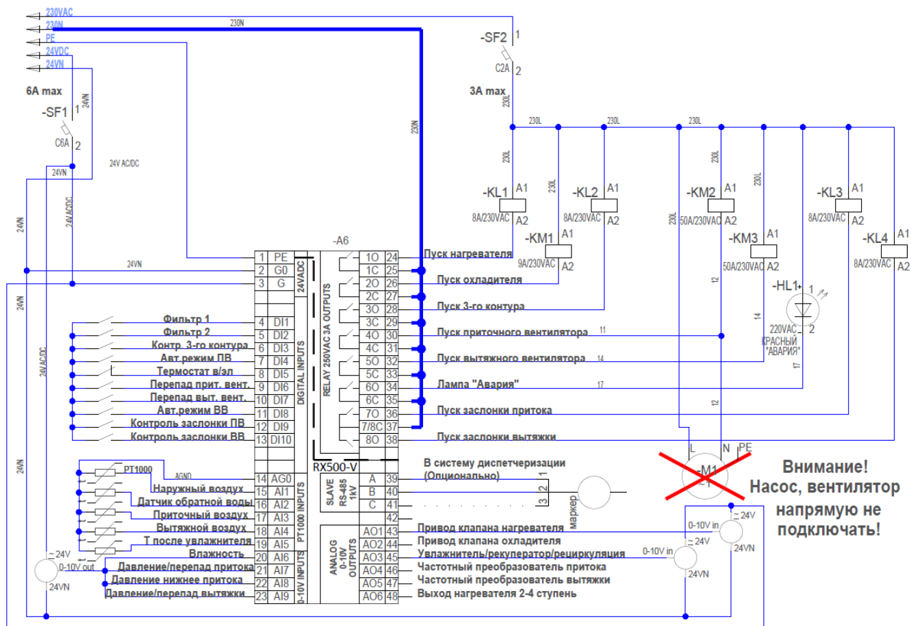
Рис.1. Схема внешних подключений к контроллеру RX500-V.
