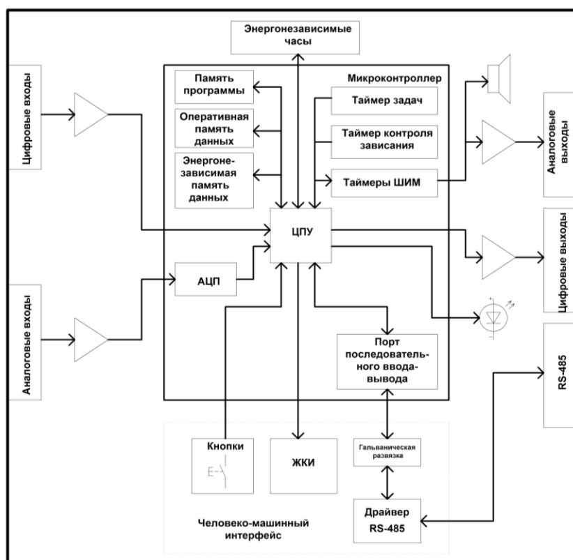
Рис.2. Аппаратная модель контроллера RX500-V.
