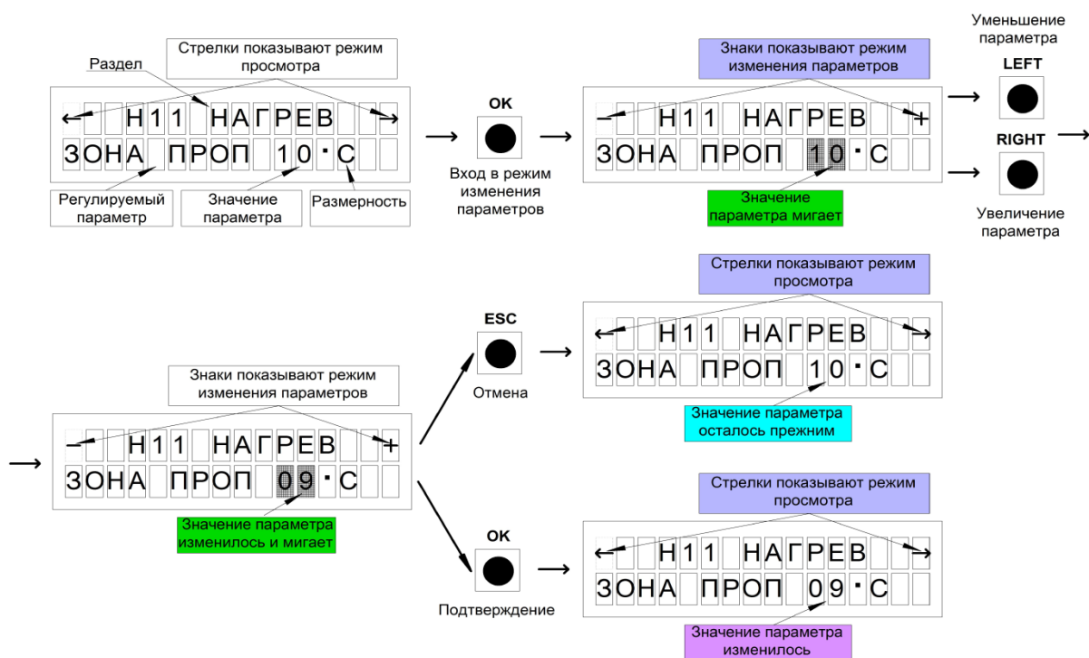
Рис. 16. Порядок изменения значения.
