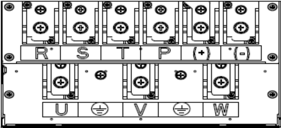
◆ 110~132кВт Силовые клеммы, 4Т модели
