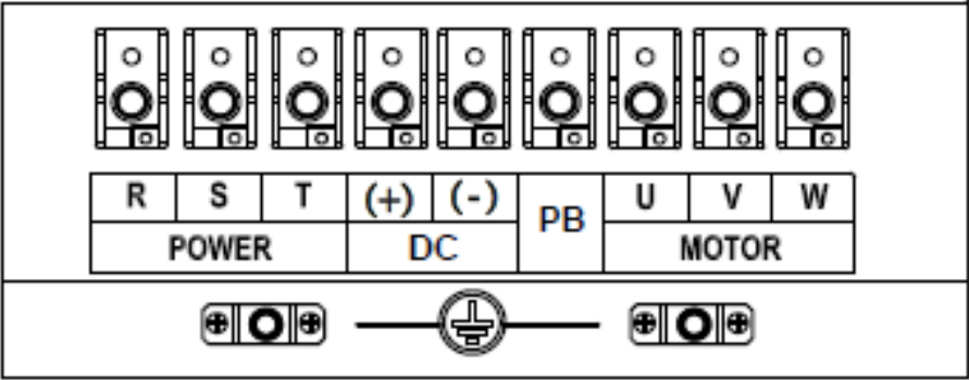
◆ 110~132кВт Силовые клеммы, 4Т модели
