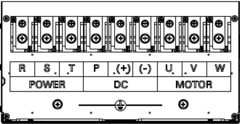
◆ 160кВт Силовые клеммы, 4Т модели
