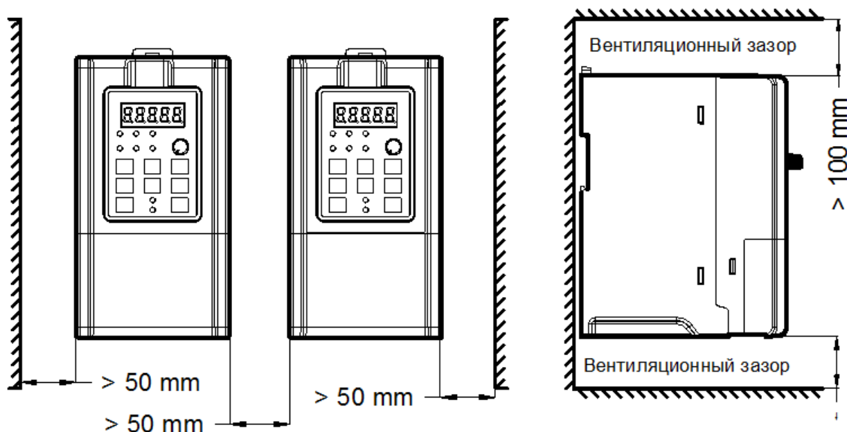
Рис. 3-1. Минимальные расстояния между ПЧ и до стенок шкафа
